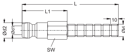
Long threaded plugs ( 060 - 090 serie ) Gewindestecker ( 060 - 090 serie )
