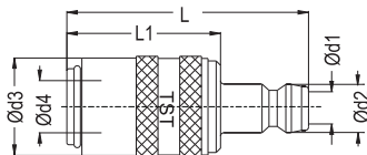
Adapting Socket with 060 - 090 Plugs Adapterkupplung mit Nippel
