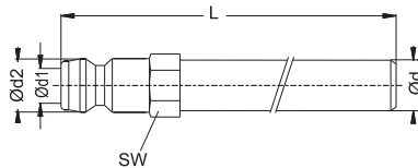
Extension Plug without thread Verlängerungsstecker ohne Gewinde
