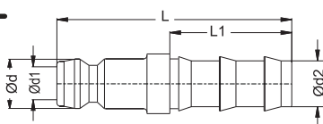
Push-Lock Hose Plug Stecknippel mit Schnellsteck - Schlauchtülle
