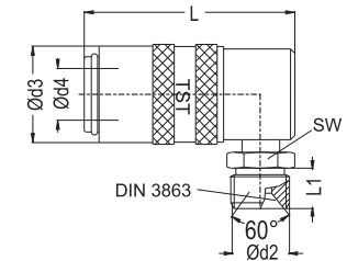
Cylindrical Male Thread socket 90° Kupplung mit 90° Aussengewinde zylindrisch
