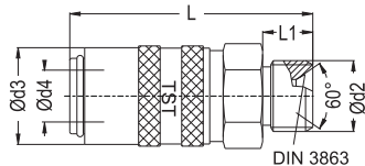
Cylindrical Male Thread socket Kupplung mit Aussengewinde zylindrisch
