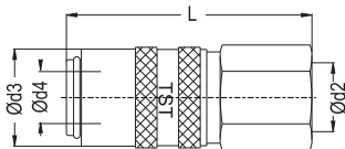
Female Thread socket Kupplung mit Innengewinde
