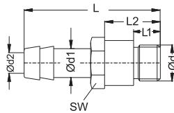
Hose nipple / Nippel mit Schlauchtülle
