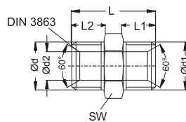
Double nipples / Doppelnippel
