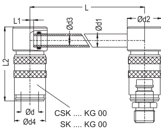
Diverting Socket / Umlenkkipplungen
