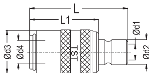
Adapting Socket With 6 - 9 Plugs Adapterkupplung mit Nippel
