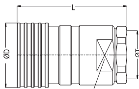
Female Thread Coupler Kupplung mit Innengewinde
