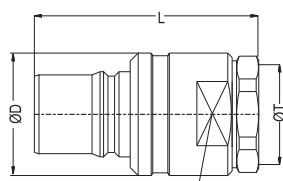
Female Thread Plug Nippel mit Innengewinde
