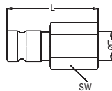
Female Threaded Shut-Off Plug Verschlussnippel mit Innengewinde
