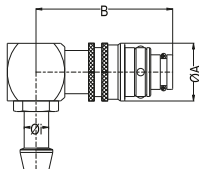
Standard hose tail plug 90° Stecker mit 90° Schlauchtülle
