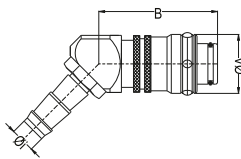
Push-lock hose tail plug 45° Stecker mit 45° Schnellsteck - Schlauchtülle
