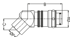
Female threaded plug 45° Stecker mit 45° Innengewinde
