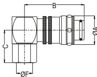
Female threaded plug 90° Stecker mit 90° Innengewinde
