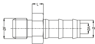
Push Lock Hose Nipple Schnellsteck - Schlauchtülle
