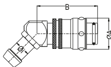
Standard hose tail plug 45° Stecker mit 45° Schlauchtülle
