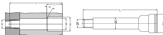
Male threaded plug socket Buchse mit Aussengewinde
