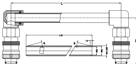
Female threaded plug 45° Stecker mit 45° Innengewinde
