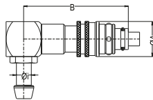
Standard hose tail plug with valve 90° Stecker mit 90° Schlauchtülle und Ventil
