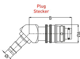
Push-lock hose tail plug 45° Stecker mit 45° Schnellsteck - Schlauchtülle
