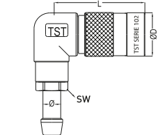
Coupler with hose tail 90° Kupplung mit 90° Schlauchtülle
