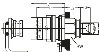
Male Threaded Socket (60° Conn. & Conn. Seating With O-ring) Kupplung mit Aussengewinde mit 60° Dichtkonus
