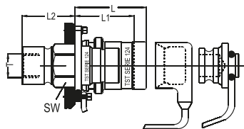
Female Threaded Socket & Plug Kupplung und Nippel mit Innengewinde
