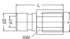
Plug with female thread Nippel mit Innengewinde
