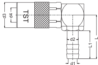
Standard hose tail socket 90° Kupplung mit 90° Standard - Schlauchtüle
