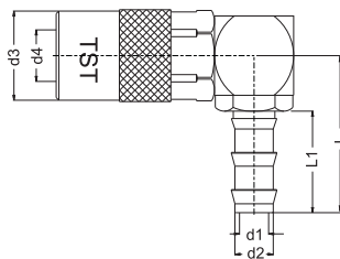
Push-Lock hose tail socket 90° Kupplung mit 90° Schnellsteck - Schlauchtülle
