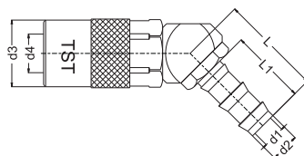
Push-Lock hose tail socket 45° Kupplung mit 45° Schnellsteck - Schlauchtüle
