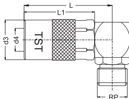
Cylindrical Thread socket 90° Kupplung mit 90° Aussengewinde zylindrisch BSP
