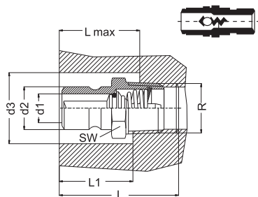
Shut-off Male threaded plug Verschlussnippel mit Außengewinde
