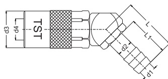
Standard hose tail socket 45° Kupplung mit 45° Schlauchtülle
