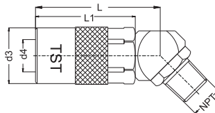
NPT Thread socket 45° Kupplung mit 45° Aussengewinde NPT
