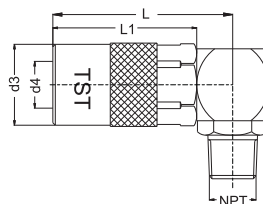
NPT Thread socket 45° Kupplung mit 90° Aussengewinde NPT
